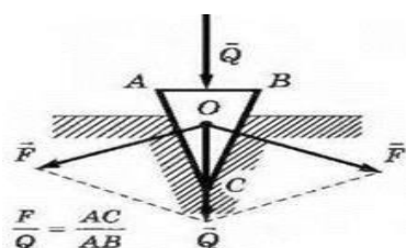
Рис. 2.6. Клин
