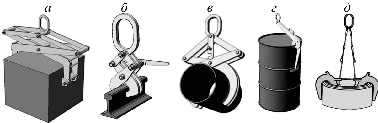
Рис. 3.33. Кліщові захвати: для бетонних блоків (а), рейок (б), труб (в), бочок (з), кілець (д)
