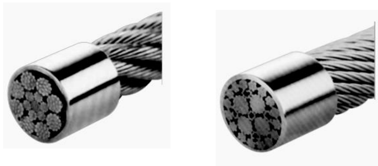
Рис. 3.2. Вантажні канати
