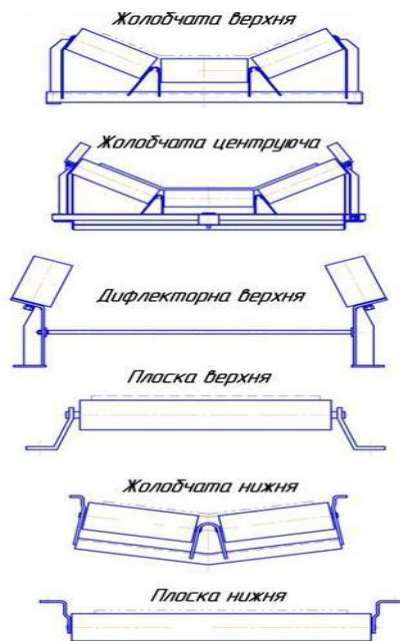
Рис. 4.19. Роликоопори
